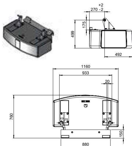
Heckgewicht 600 & 900 kg
