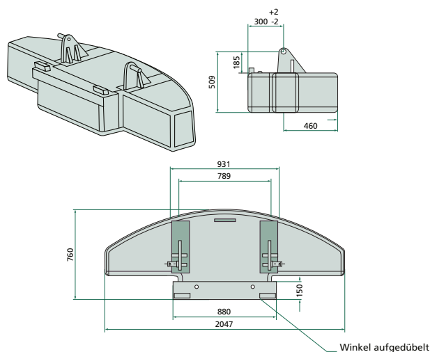
Heckgewicht 1250 & 1450 kg
